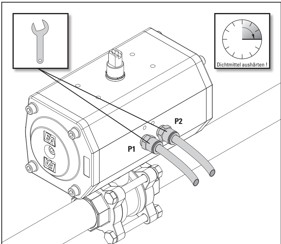
Abb. 7.4 - Montage / Demontage, Pneumatische Installation Funktion doppeltwirkend
