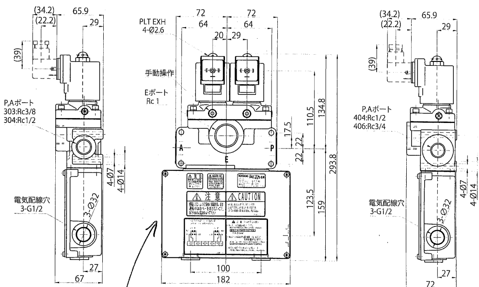
■ AD-SL231D-404E,406E-M2(K)-D※
