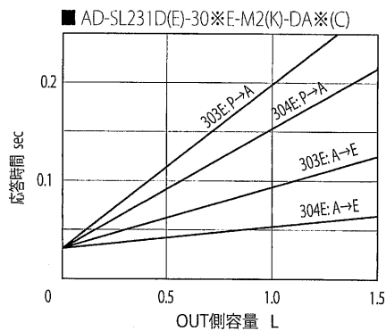
■ AD-SL231D-303E,304E-M2(K)-D※
