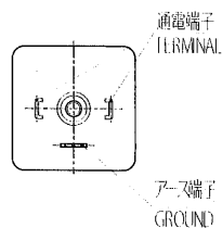
DINコネクタ配線図 DIN CONNECTOR WIRING
