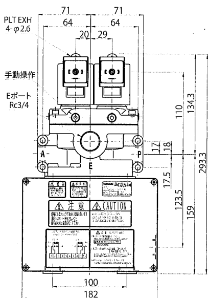
■ AD-SL231D-303E,304E-M2(K)-D※
