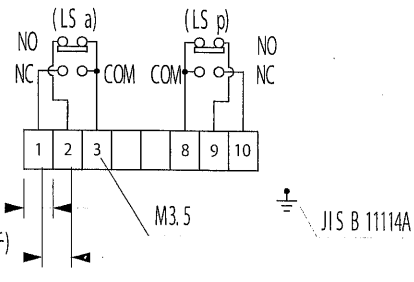
端子台配線図 TERMINAL WIRING
