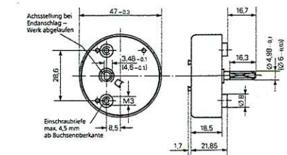
ohne Kontakte
