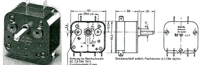
ohne Rastung
