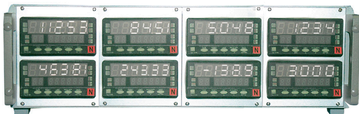
Frontansicht: Bis zu 8 Anzeiger in einem 19"-84TE-Gehäuse möglich.
