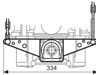
Attacco rapido 1"3/8 F. Quick coupler 1"3/8 F. Enganche 3 puntos toma de fuerza H. 1"3/8 Prise rapide 1"3/8 F. 3-Punkt Schnellanschluß 1"3/8 mit Ketten
