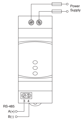
CEM-M-RS-485
